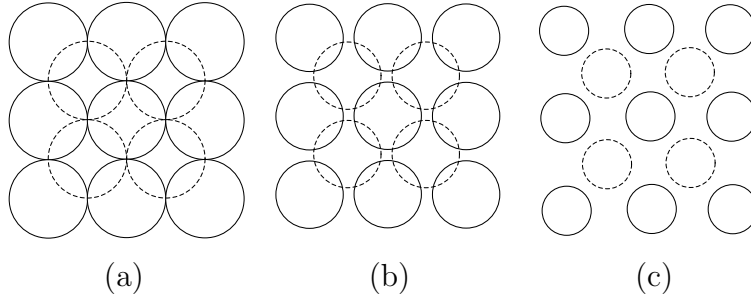
Figure 5.6: Illustration schématique des trois situations possibles dans le modèle simple de sphères.
