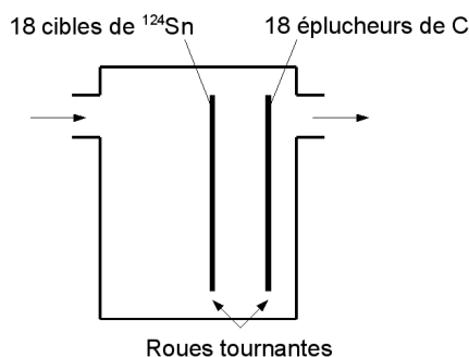
FIGURE 4.12: Schéma de la chambre à réaction FULIS. Cette dernière est composée de deux roues de rayon 36 cm destinées à accueillir 18 cibles et 18 éplucheurs de Carbone. Les roues effectuent (jusqu'à) 2000 rotations par minute afin de ne pas dégrader les cibles et rester en dessous de leur point de fusion.
