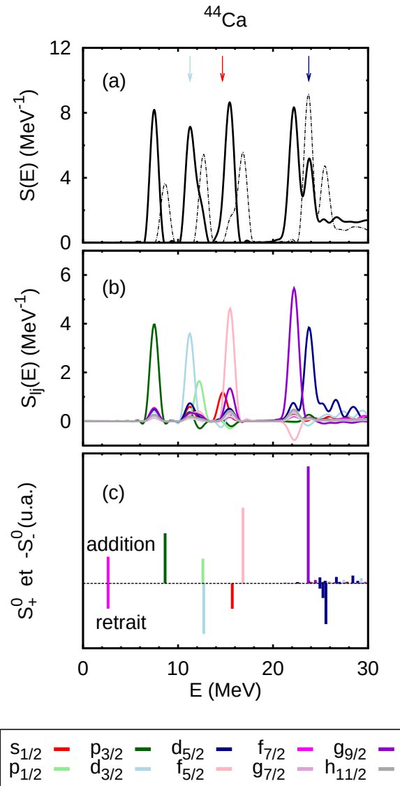
FIGURE 3.6: (a) : Distribution de force S(E) de l'opérateur \hat{F} du ^{44}\text{Ca} (en traits plein) et son équivalent non perturbé ( S^0(E) ) (traits pointillés). (b) : Distribution de force décomposée selon ses contributions en termes de nombres quantiques de quasiparticule S_{ij} . Chaque nombre quantique est associé à une couleur, indiquée dans la légende. (c) : Spectre non perturbé des opérateurs ajout S_+^0(E) et retrait de paire de nucléons -S_-^0(E) indiqué en échelle négative. Ces derniers servent à discriminer les modes de type ajout ou retrait de paires de nucléons. Les flèches au dessus de certains pics du panneau (a) correspondent aux modes de retrait (excitations du noyau A - 2 ).
