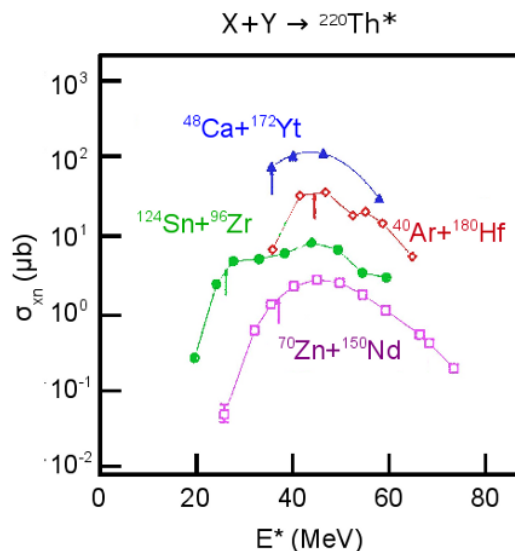
FIGURE 4.2: Sections efficaces de fusion-évaporation passant par la formation du noyau composé de ^{220}\text{Th}^* , obtenu avec différents partenaires de collision ( ^{124}\text{Sn} + ^{96}\text{Zr} [Sah85], ^{172}\text{Yb} + ^{48}\text{Ca} [Sah85], ^{180}\text{Hf} + ^{40}\text{Ar} [Ver84] et ^{150}\text{Nd} + ^{70}\text{Zn} [Sto98]). Cette figure est extraite de [Sto98].
