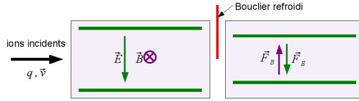
FIGURE 4.13: Schéma du filtre de Wien de la ligne LISE3. Séparé en deux sections par un bouclier refroidi destiné à stopper le faisceau incident, il est le siège d'une combinaison de champ électrique et magnétique orthogonaux dont l'action est de laisser passer les ions de vitesse considérée en bloquant les autres, notamment les ions du faisceau incident. Les distances entre les plaques électrostatiques du filtre de Wien de LISE3 n'étaient pas les mêmes dans les deux sections, mais les potentiels appliqués étaient destinés à y créer le même champ électrique.
