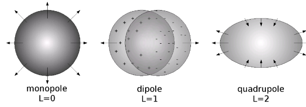
FIGURE 2.1: Représentation schématisée des résonances géantes monopolaire ( L=0, S=0, T=0 ), dipolaire ( L=1, S=0, T=1 ), et quadrupolaire ( L=2, S=0, T=0 ).
